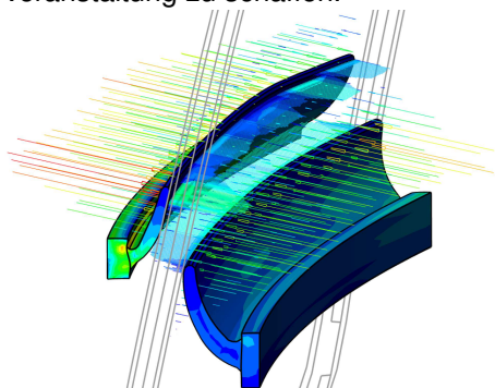
Fensterdichtung (Tmeet2021)
